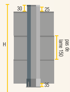
Assemblage Ranch tablier plein PB09 (100)
