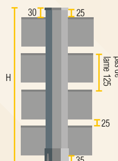
Assemblage Brise vue CL07 (136)
