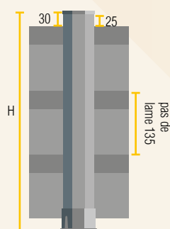
Assemblage Brise vue CL07 (136)
