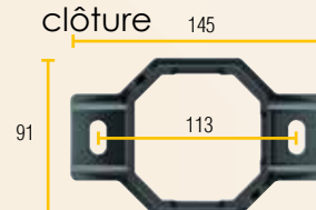
ST3603A (pied) support de fixation pour poteau de clôture
