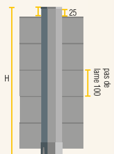
Assemblage Ranch tablier plein PB09 (100)
