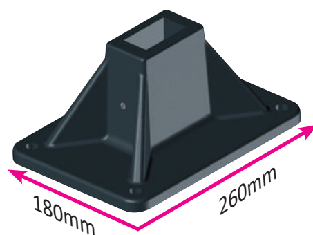
Platine de fixation ST24
