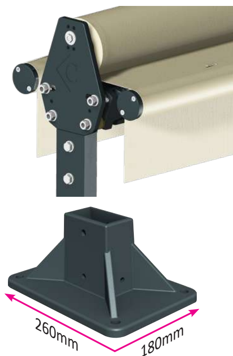
Platine de fixation ST10
