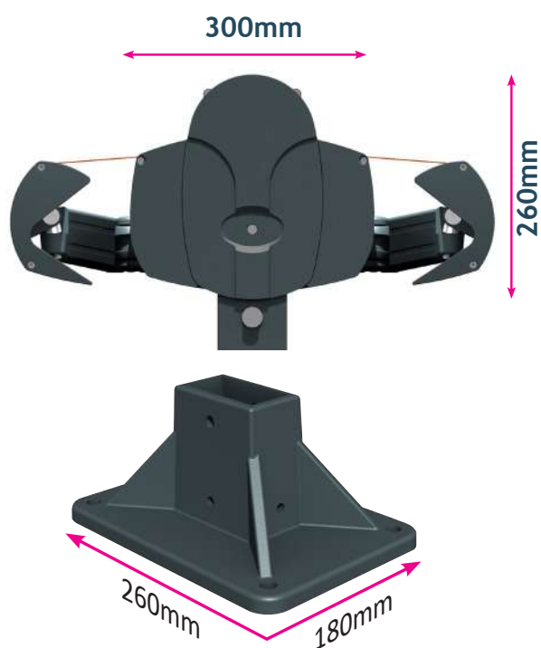
Platine de fixation ST10
