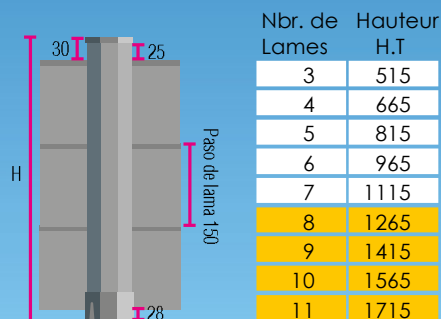
Montaje Ranch sin visibilidad PB06 (150)
