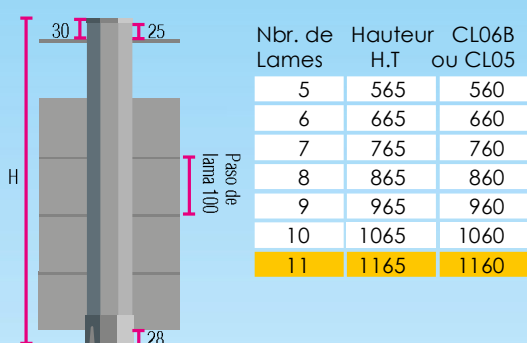
Montaje Ranch sin visibilidad PB09 (100)
