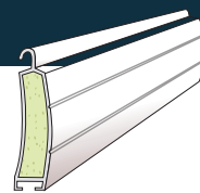
Espuma aislante
