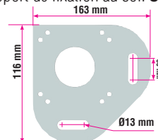
Support de fixation au sol: ST4502
