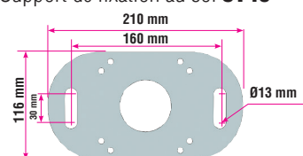
Support de fixation au sol ST45
