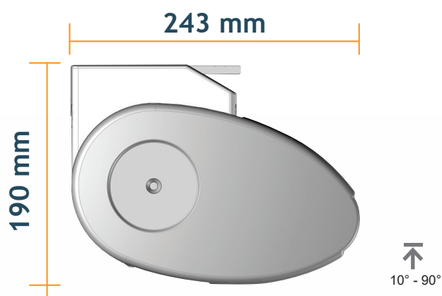
Encombre Support Plafond
