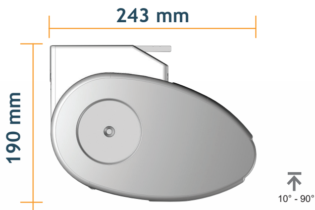
Dimensiones Soporte de techo
