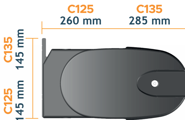
Dimensiones del soporte de pared
